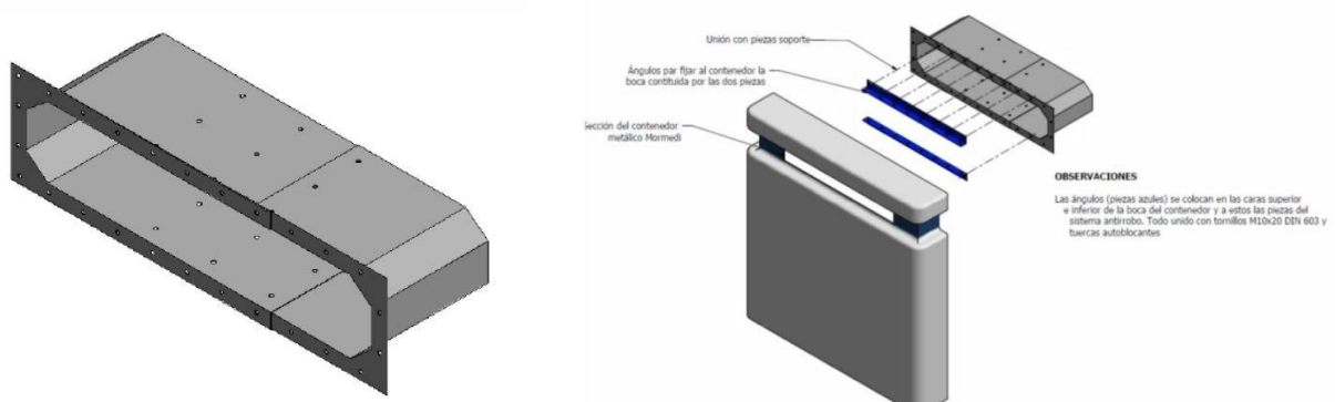
Figura 1. Exemple de sistema per dificultar el robatori del paper-cartró en contenidors de càrrega superior (l/lI): allargament cap a dins de la boca d'entrada amb la instal·lació d'una xapa amb angle recte al contenidor.
